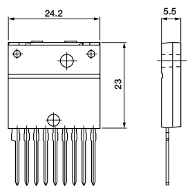
STR-S
