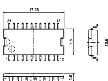
SPF24pin
