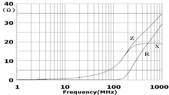
FBU201209T-170Y-S
