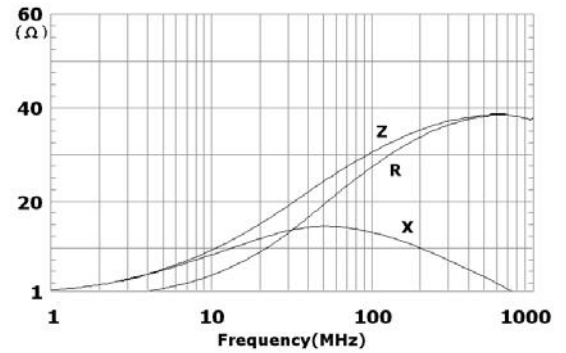
FBU201209T-600Y-S
