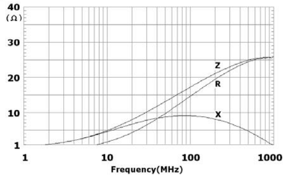
FBU201209T-390Y-S
