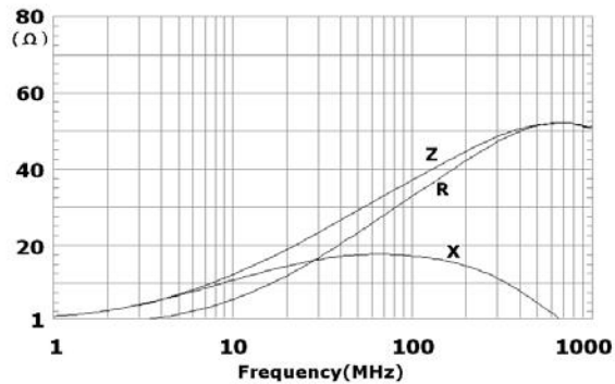
FBU201209T-800Y-S
