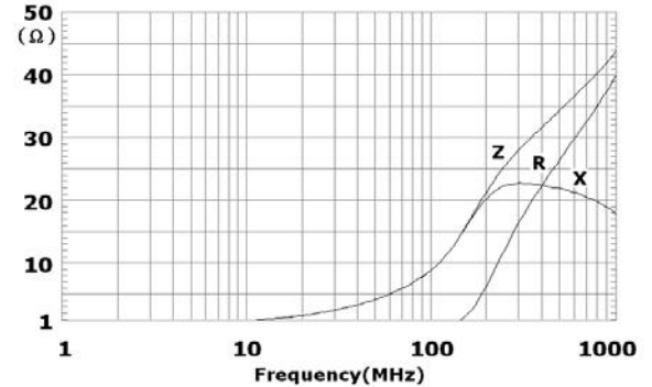
FBU201209T-300Y-S
