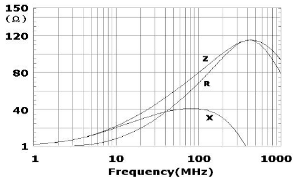
FBU201209T-800Y-S
