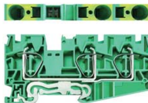
DST 16/3-PE-D
