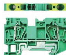
DST 6-PE-D
