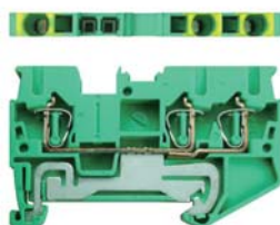
DST 2.5/3-PE-D
